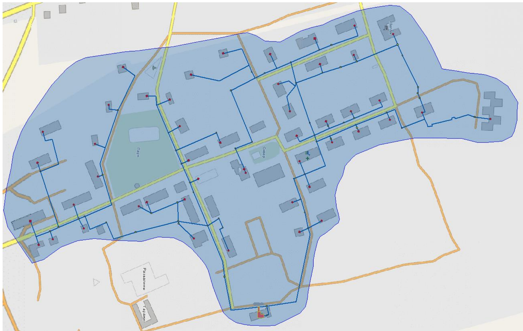
Рисунок 1.20. Зона действия котельной №11 пос. Кобринское
