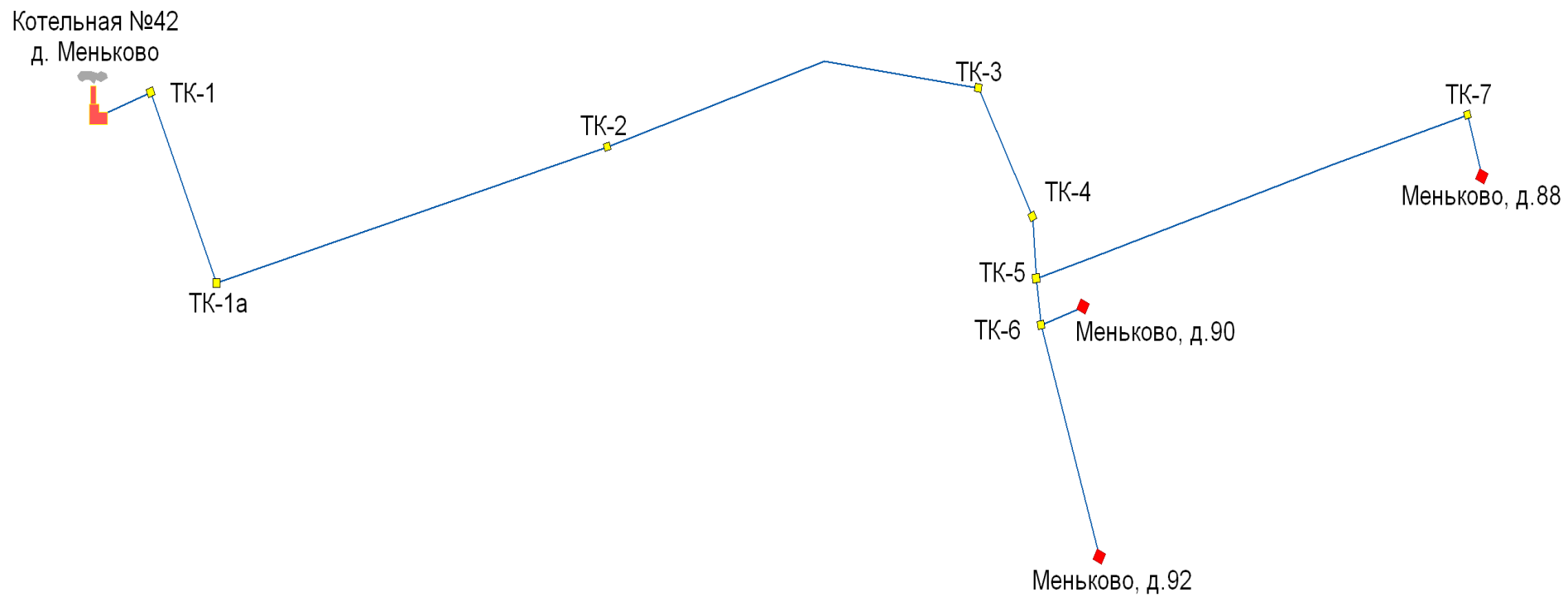
Рисунок 1.12. Схема тепловых сетей котельной №42 дер. Меньково (контур ГВС)
