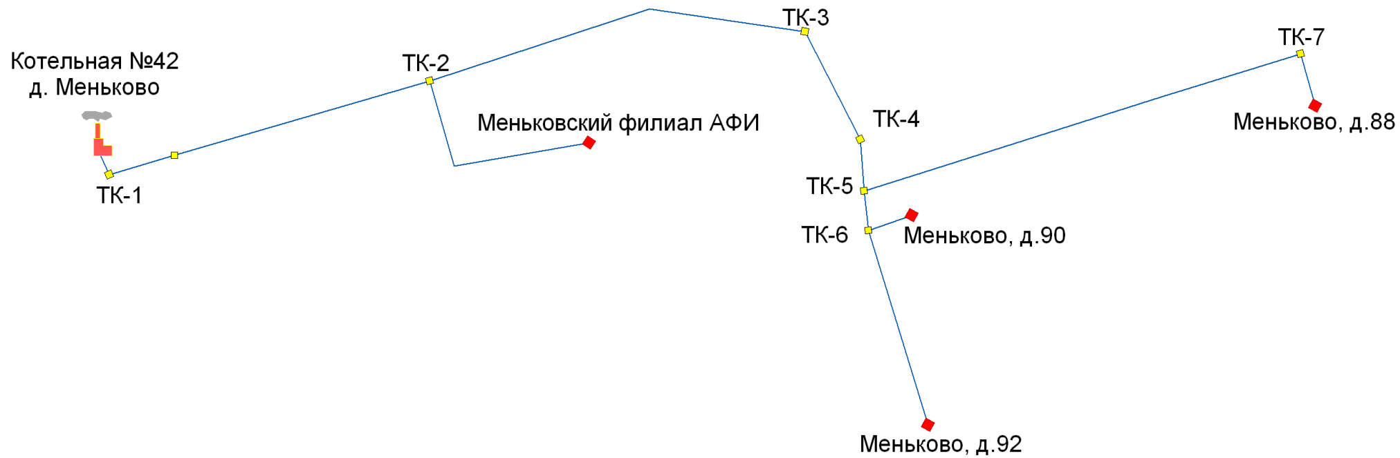
Рисунок 1.11. Схема тепловых сетей котельной №42 дер. Меньково (контур отопления)
