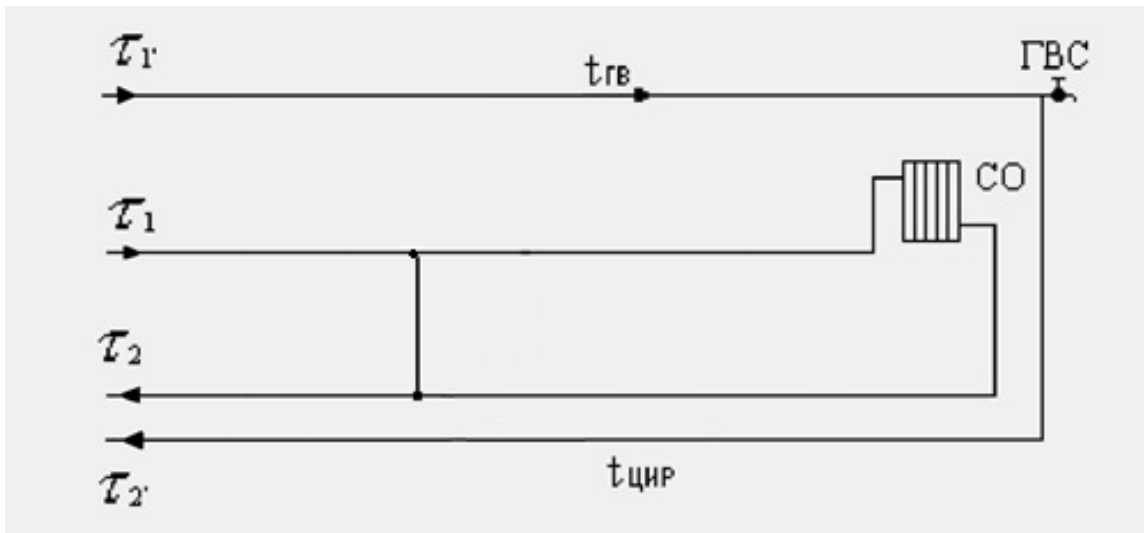
Рисунок 1.18. Схема подключения потребителей к четырехтрубным системам теплоснабжения
