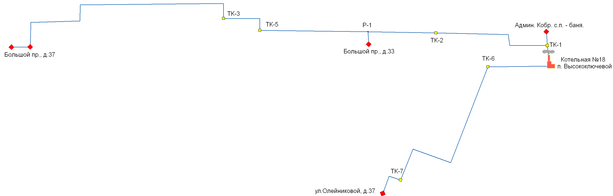
Рисунок 1.10. Схема тепловых сетей котельной №18 пос. Высокоключевой (контур ГВС)
