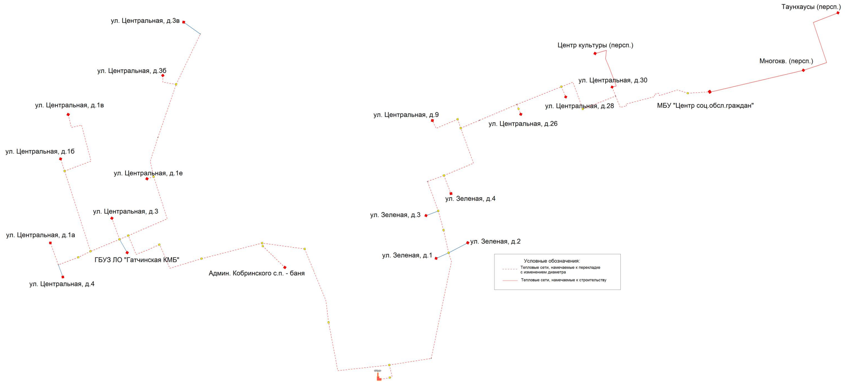
Рисунок 4.6. Схемы тепловых сетей котельной №11 пос. Кобринское на 2030 год (контур ГВС)
