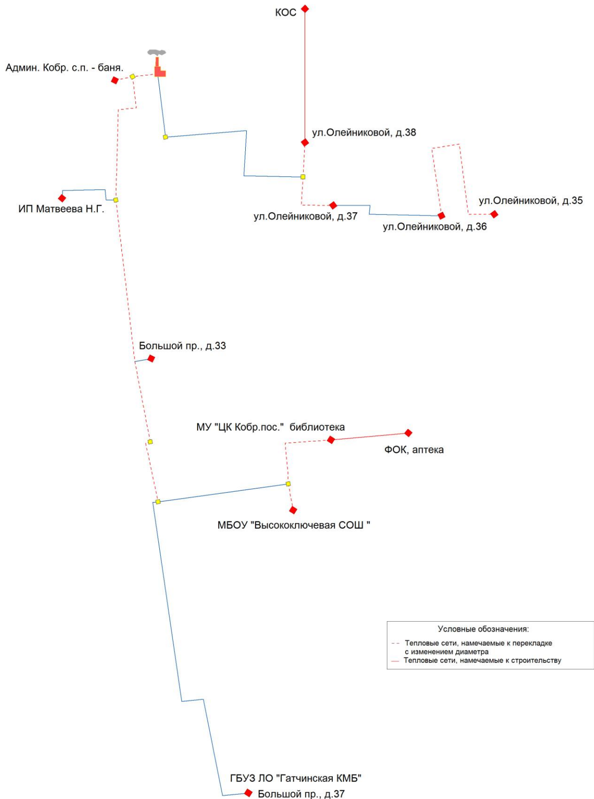
Рисунок 4.8. Схемы тепловых сетей котельной №18 пос. Высокоключевой на 2030 год (контур отопления)
