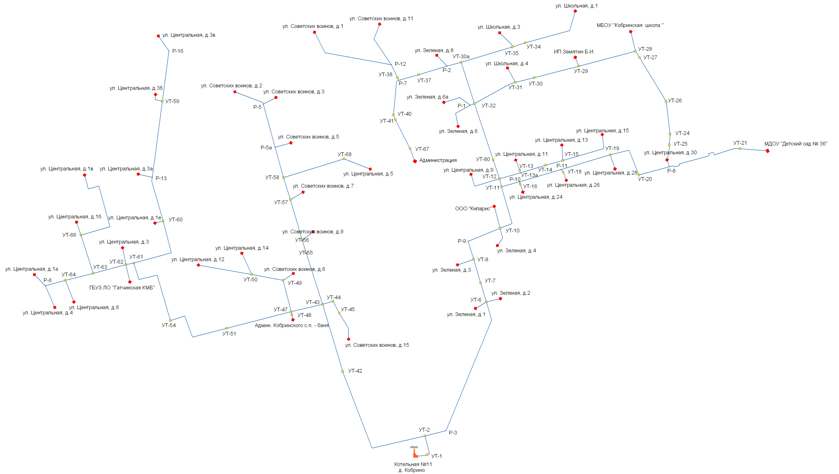
Рисунок 1.6. Схема тепловых сетей котельной №11 пос. Кобринское (контур отопления)
