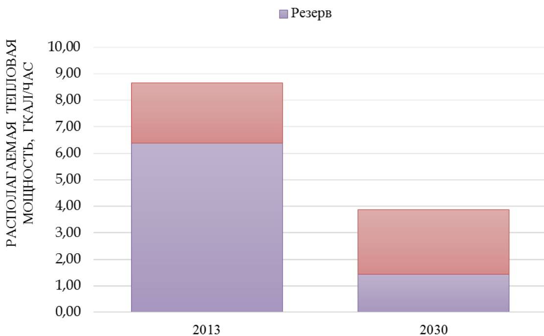
Рисунок 4.2. Балансы тепловой мощности и перспективной тепловой нагрузки котельной №17 пос. Суйда
