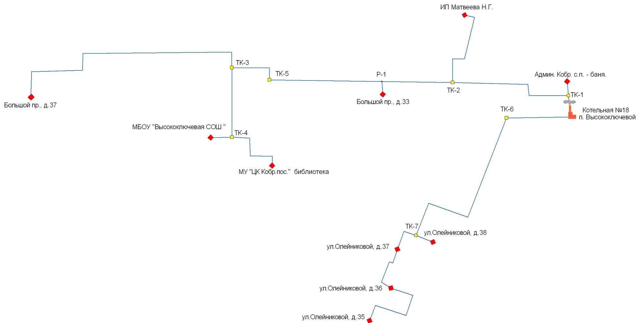
Рисунок 1.9. Схема тепловых сетей котельной №18 пос. Высокоключевой (контур отопления)
