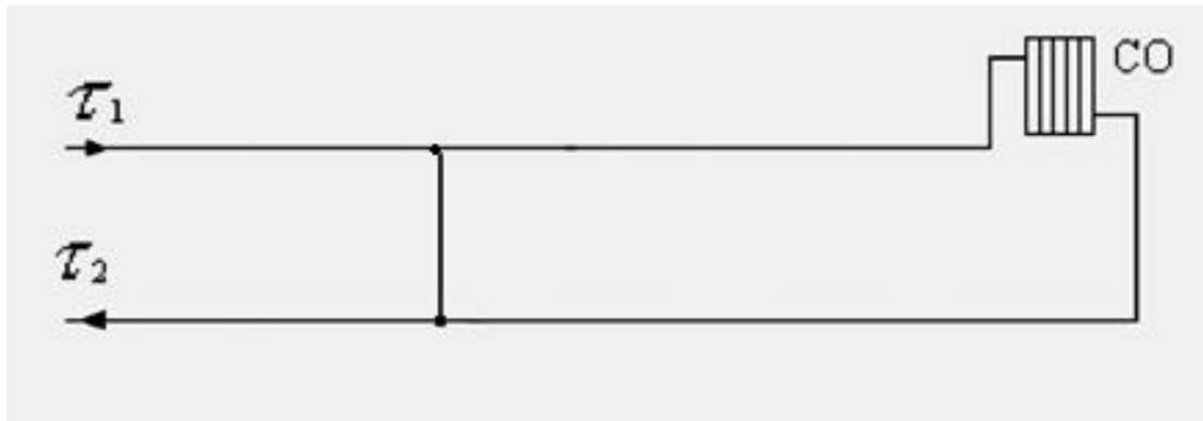
Рисунок 1.19. Схема подключения потребителей к двухтрубным системам теплоснабжения
