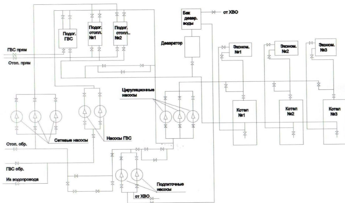
Рисунок 1.2. Тепловая схема котельной №11 пос. Кобринское
