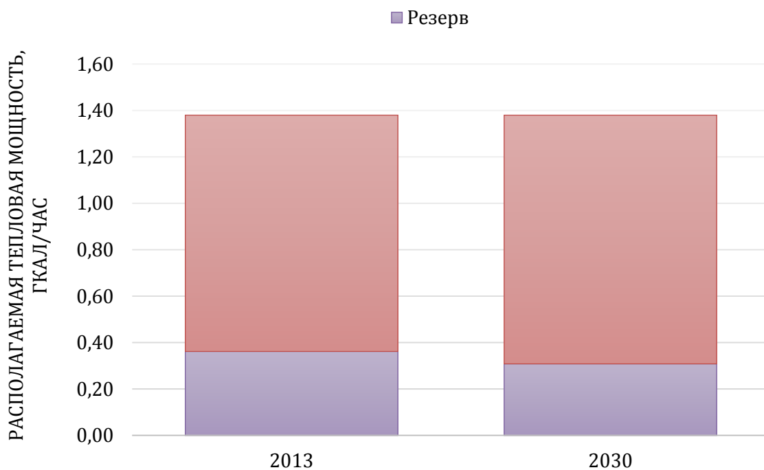
Рисунок 4.4. Балансы тепловой мощности и перспективной тепловой нагрузки котельной №42 дер. Меньково
