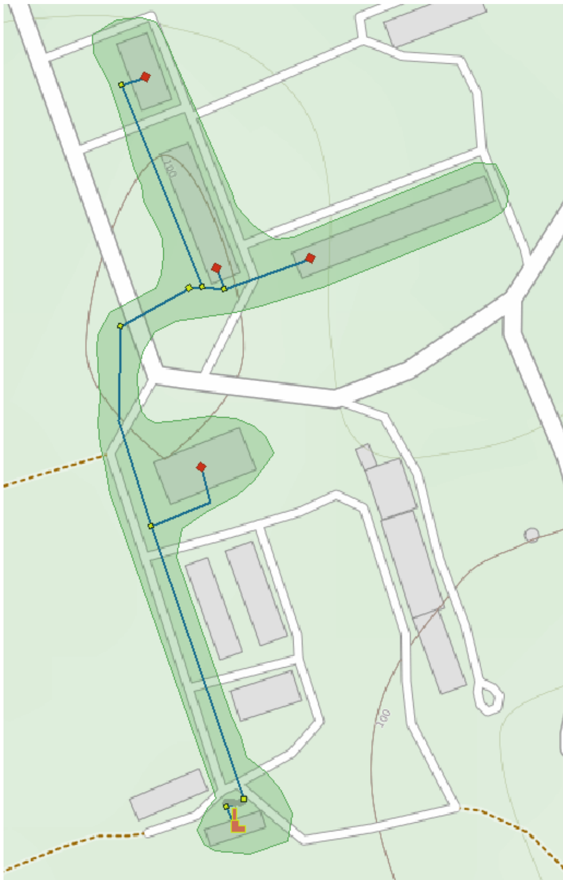
Рисунок 1.23. Зона действия котельной №42 дер. Меньково
