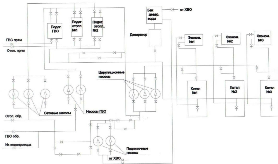
Рисунок 1.4. Тепловая схема котельной №18 пос. Высокоключевой.
