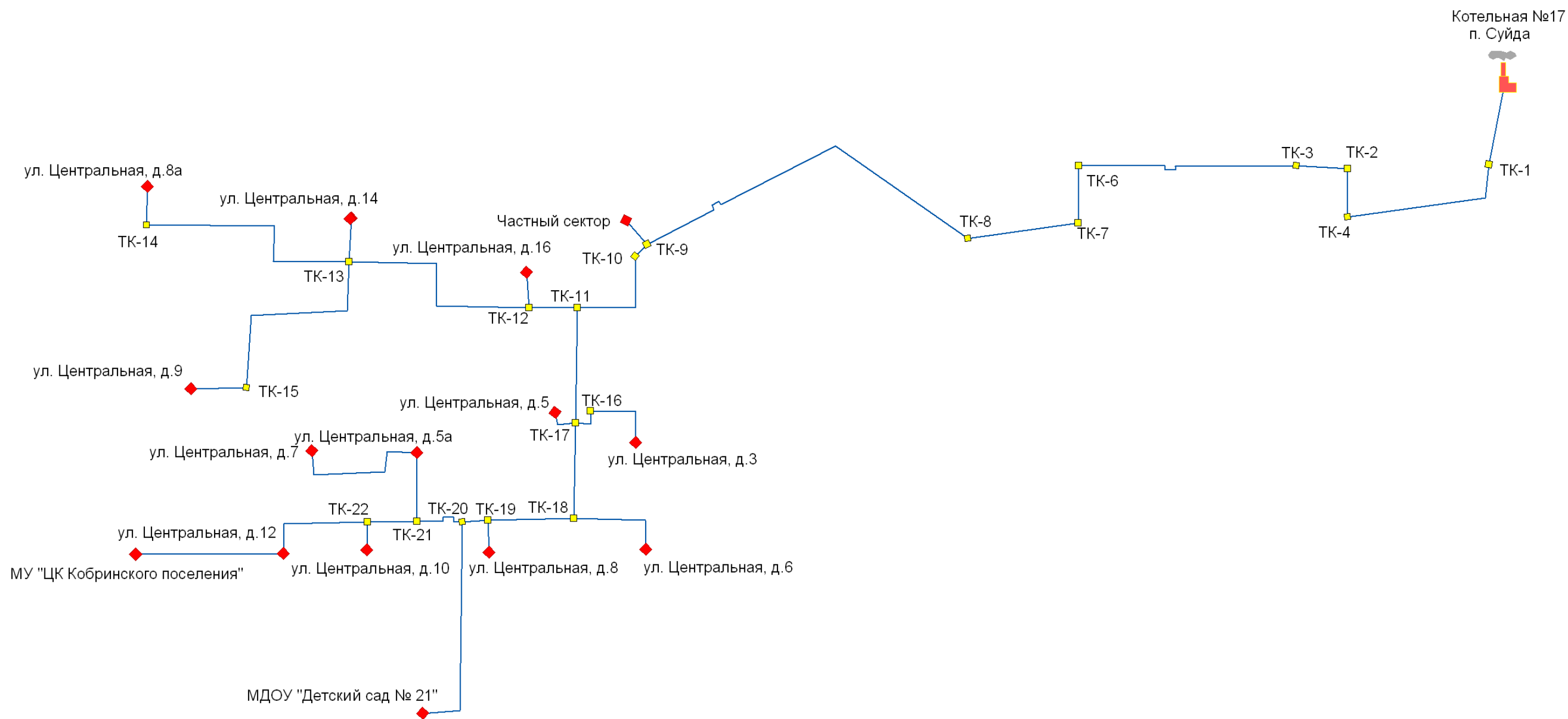
Рисунок 1.8. Схема тепловых сетей котельной №17 пос. Суйда
