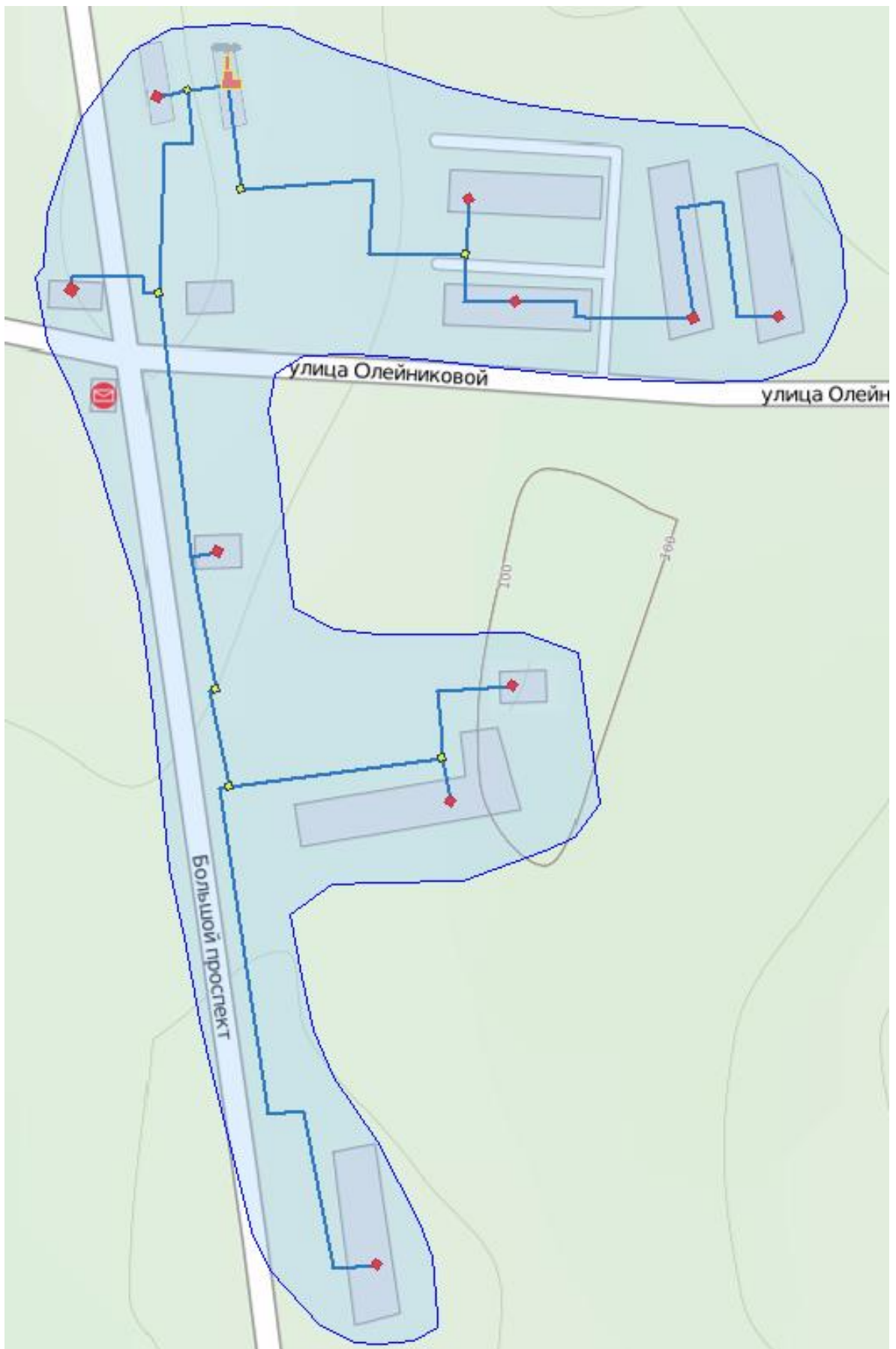
Рисунок 1.22. Зона действия котельной №18 пос. Высокоключевой
