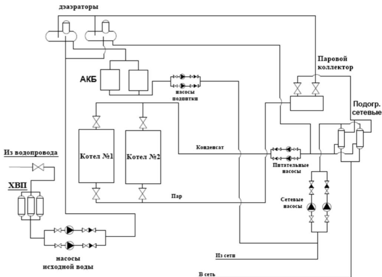
Рисунок 1.3. Тепловая схема котельной №17 пос. Суйда
