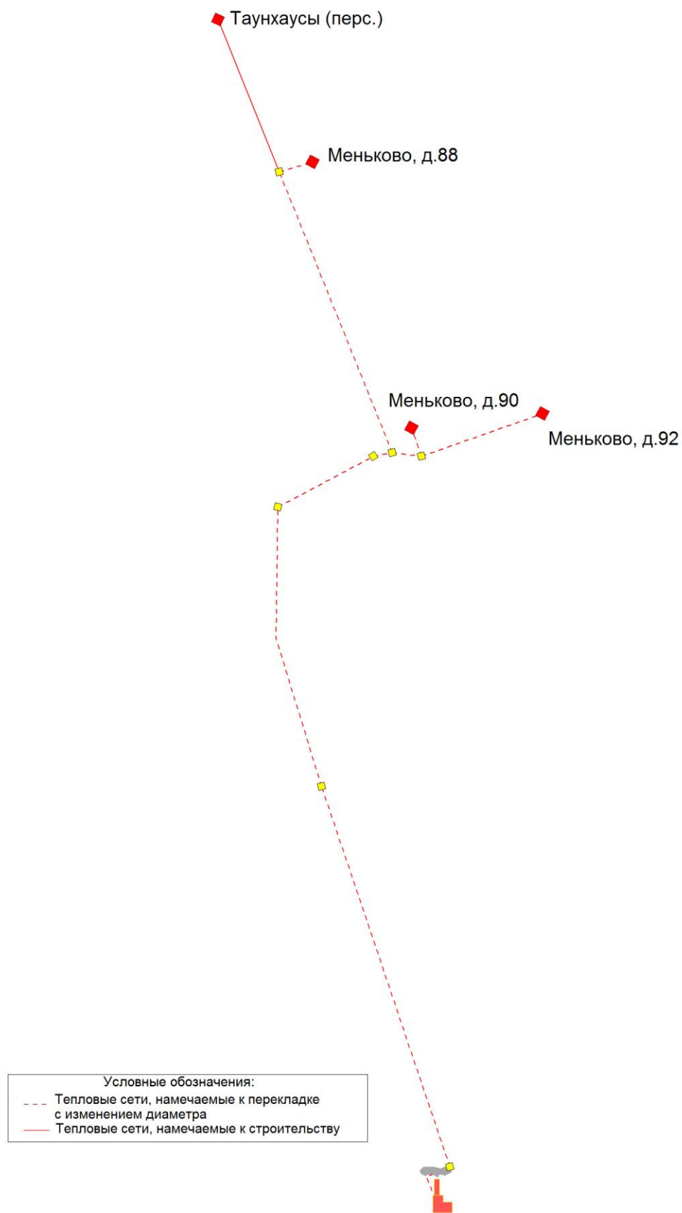
Рисунок 4.11. Схемы тепловых сетей котельной №42 дер. Меньково на 2030 год (контур ГВС)
