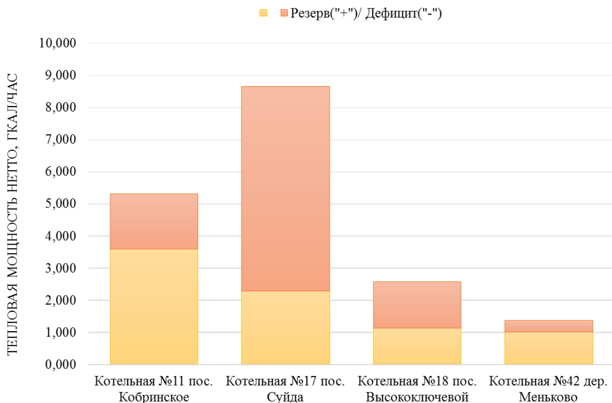
Рисунок 1.25. Резервы и дефициты тепловой мощности нетто источников централизованного теплоснабжения на территории Кобринского сельского поселения
