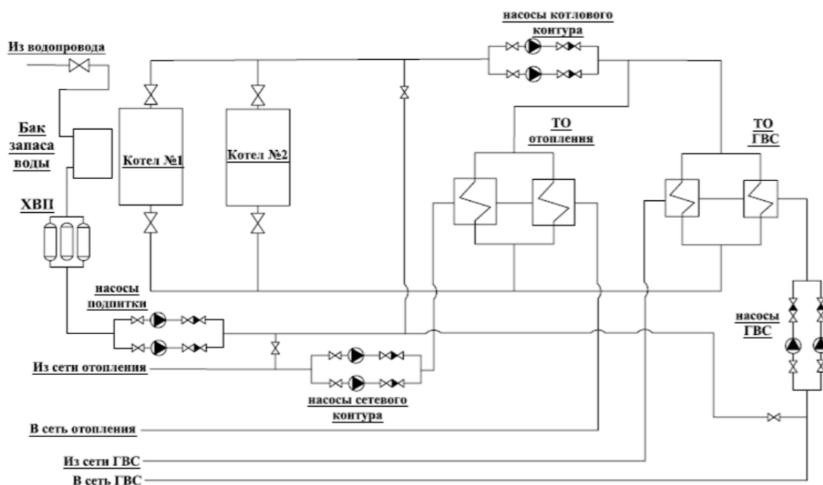
Рисунок 1.5. Тепловая схема котельной №42 дер. Меньково
