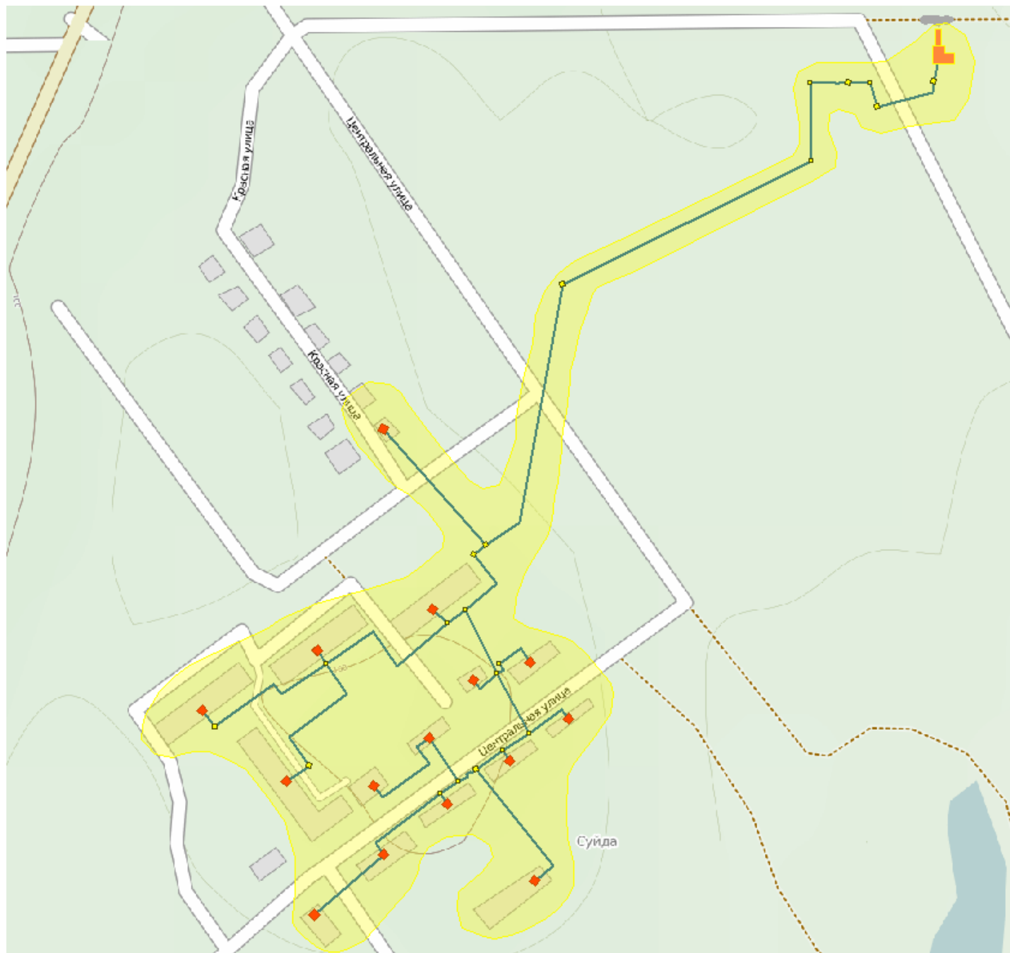
Рисунок 1.21. Зона действия котельной №17 пос. Суйда
